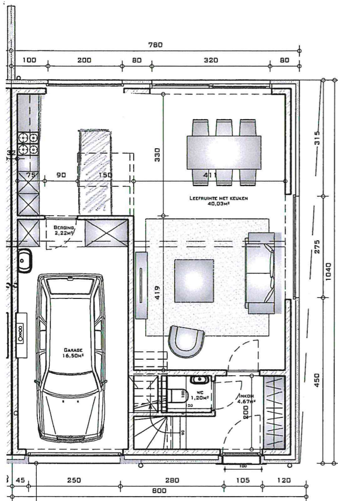
WONING LOT B GELIJKVLOERS
