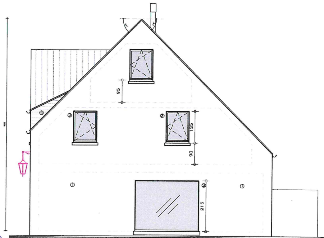
WONING LOT B ZIJGEVEL RECHTS
