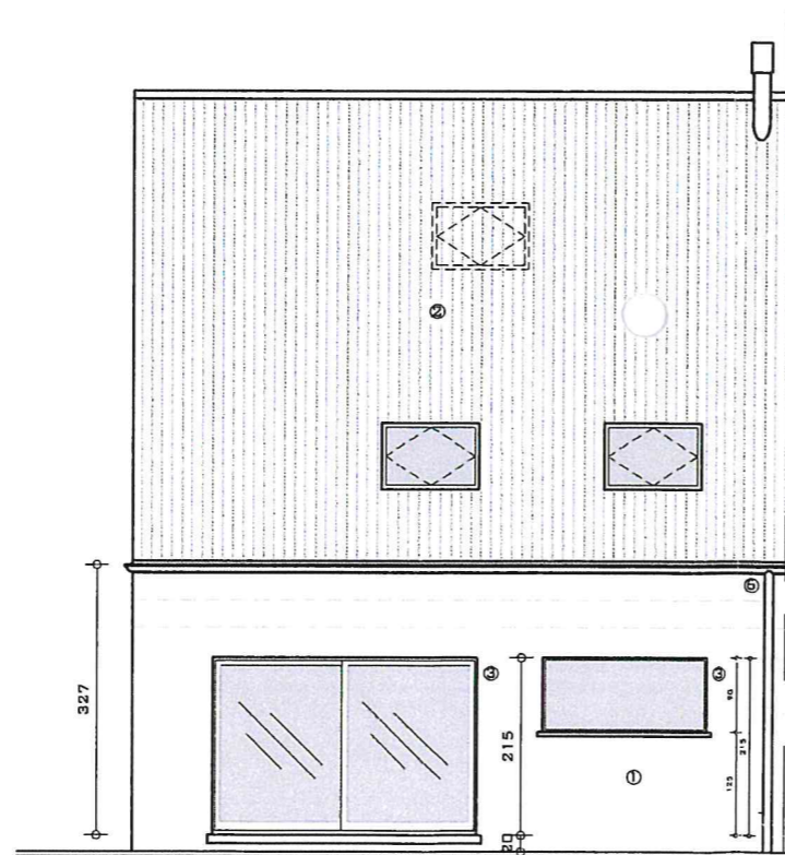
WONING LOT B ACHTERGEVEL
